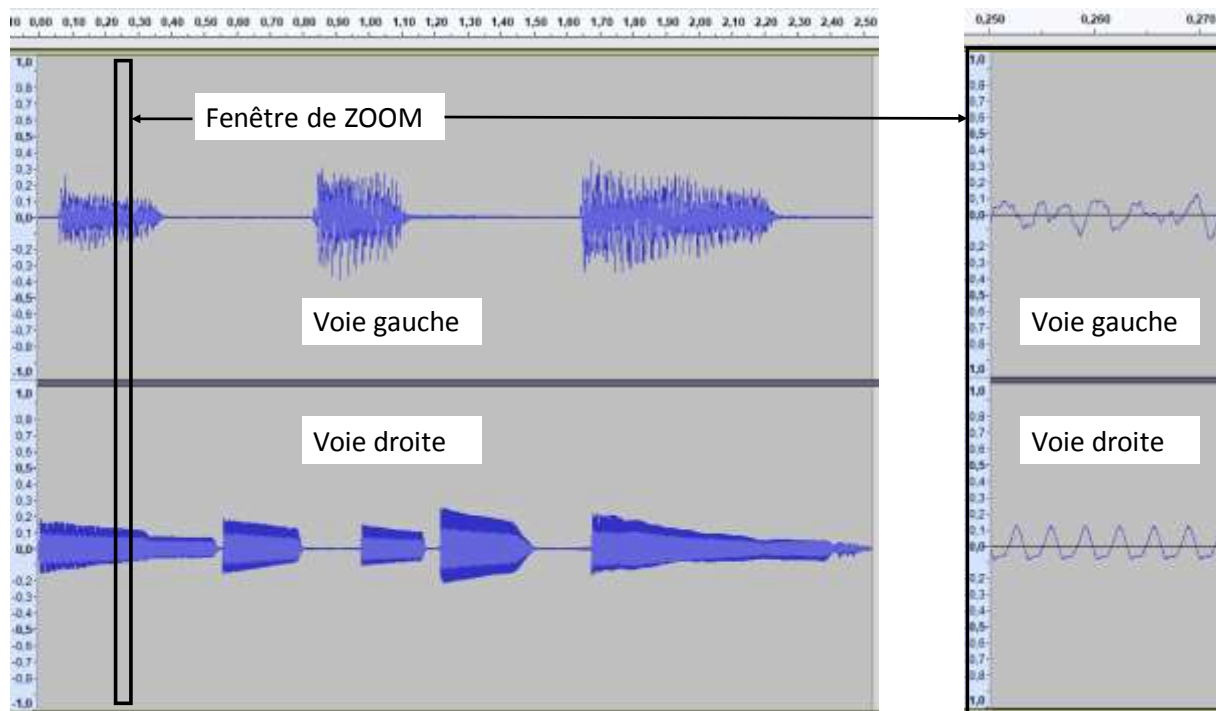
Figure 8 : Signal audio numérique stéréo
