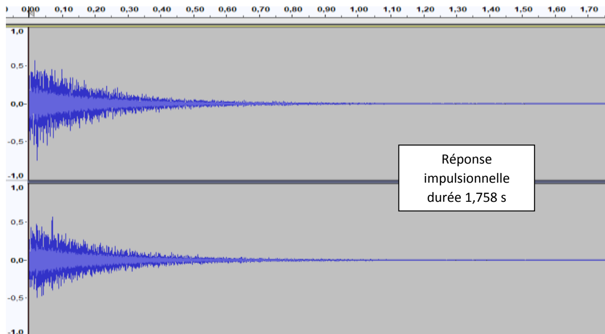
Figure 12 : réponse impulsionnelle
