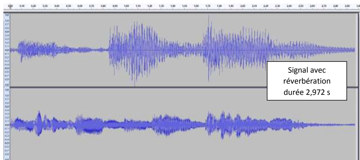
Figure 13 : signal avec réverbération
